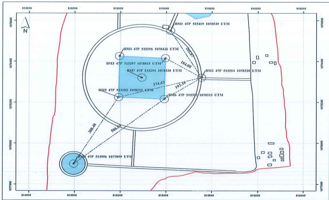
ภาพที่ 12 แสดงผังการผังแบบการขุดบ่อ A1 พื้นที่ 14 ไร่
