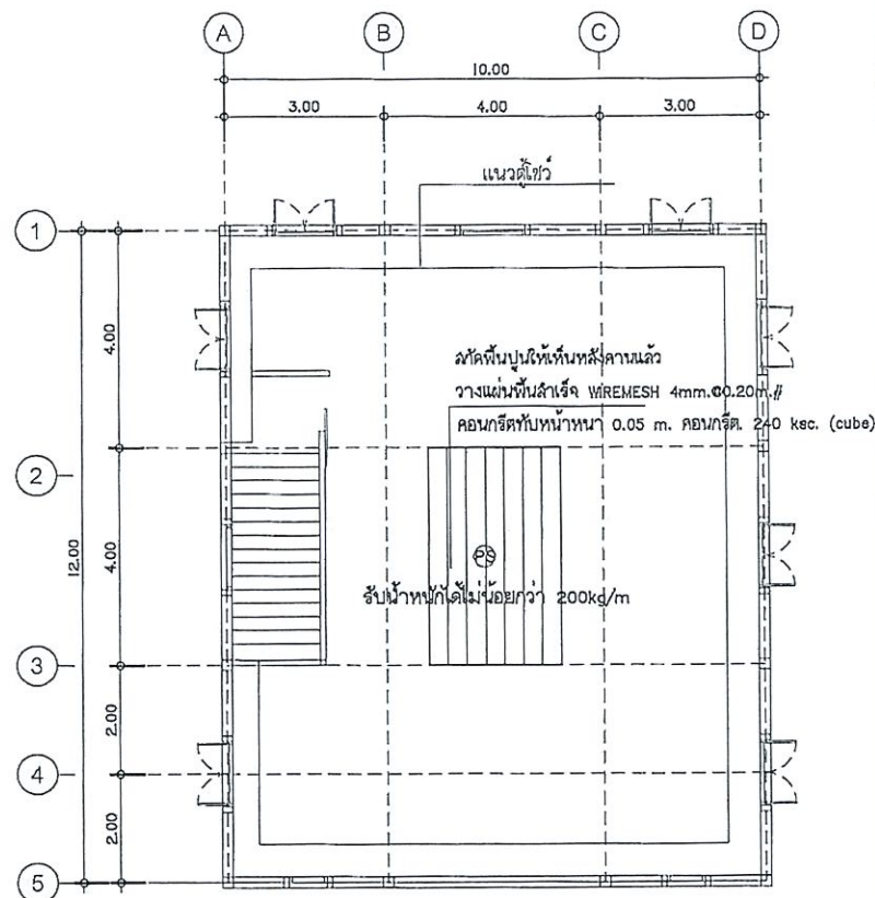
แบบแสดง แปลนโครงสร้างชั้น 2
