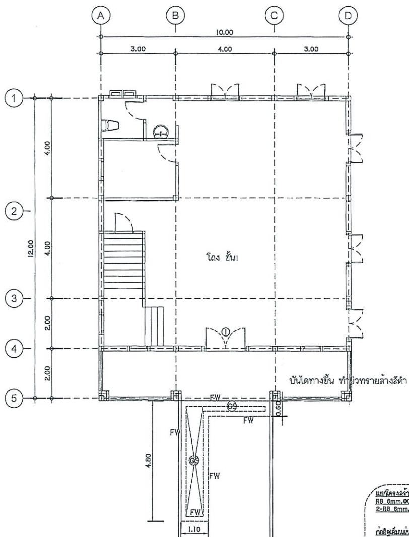
แบบแสดง แปลนโครงสร้างชั้น 1
