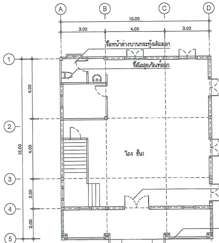
แบบแสดง แปลนพื้นชั้น1 ก่อนปรับปรุง
