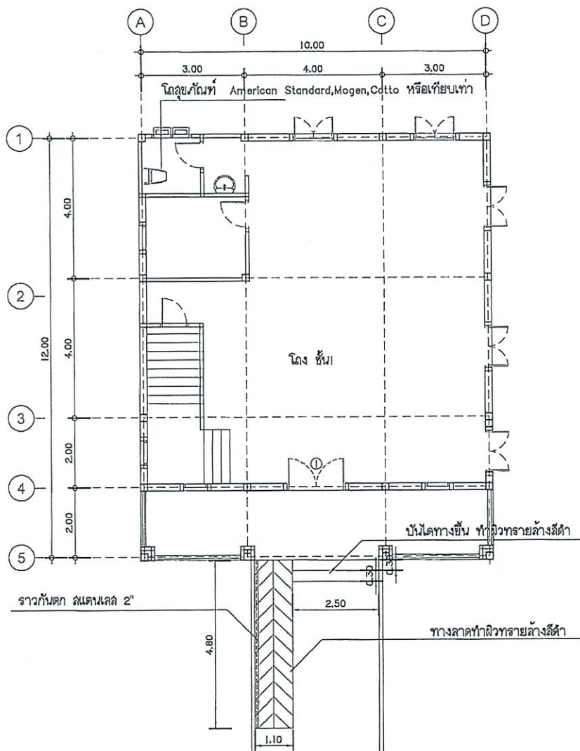
แบบแสดง แปลนพื้นชั้น 1
