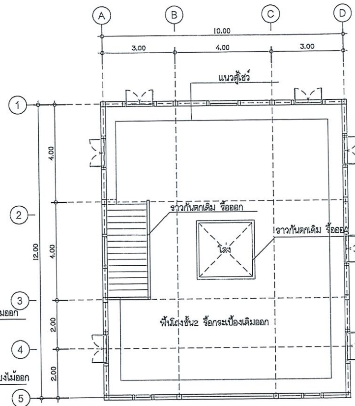
แบบแสดง แปลนพื้นชั้น2 ก่อนปรับปรุง
