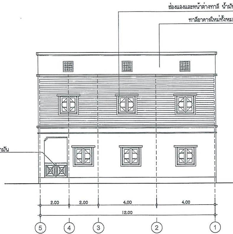
แบบแสดง ภูมิด้านข้างขวา มาตราส่วน 1 : 100
