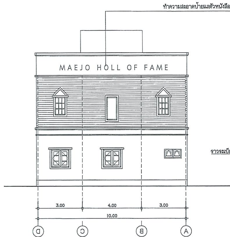
แบบแสดง ภูมิด้านหลัง มาตราส่วน 1 : 100
