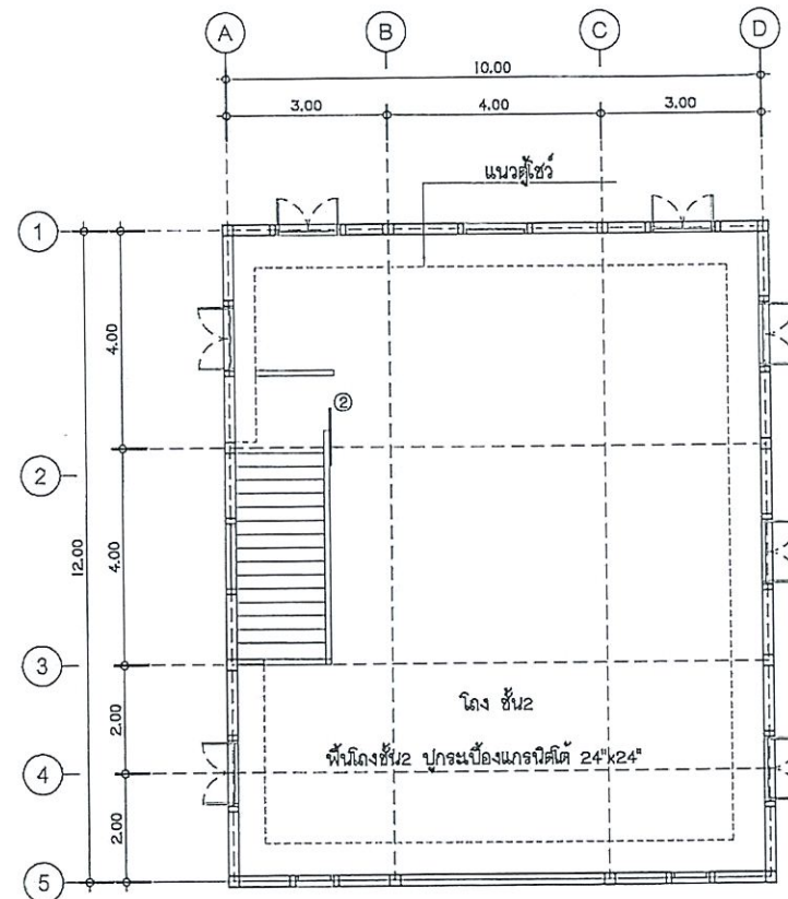
แบบแสดง แปลนพื้นชั้น 2
