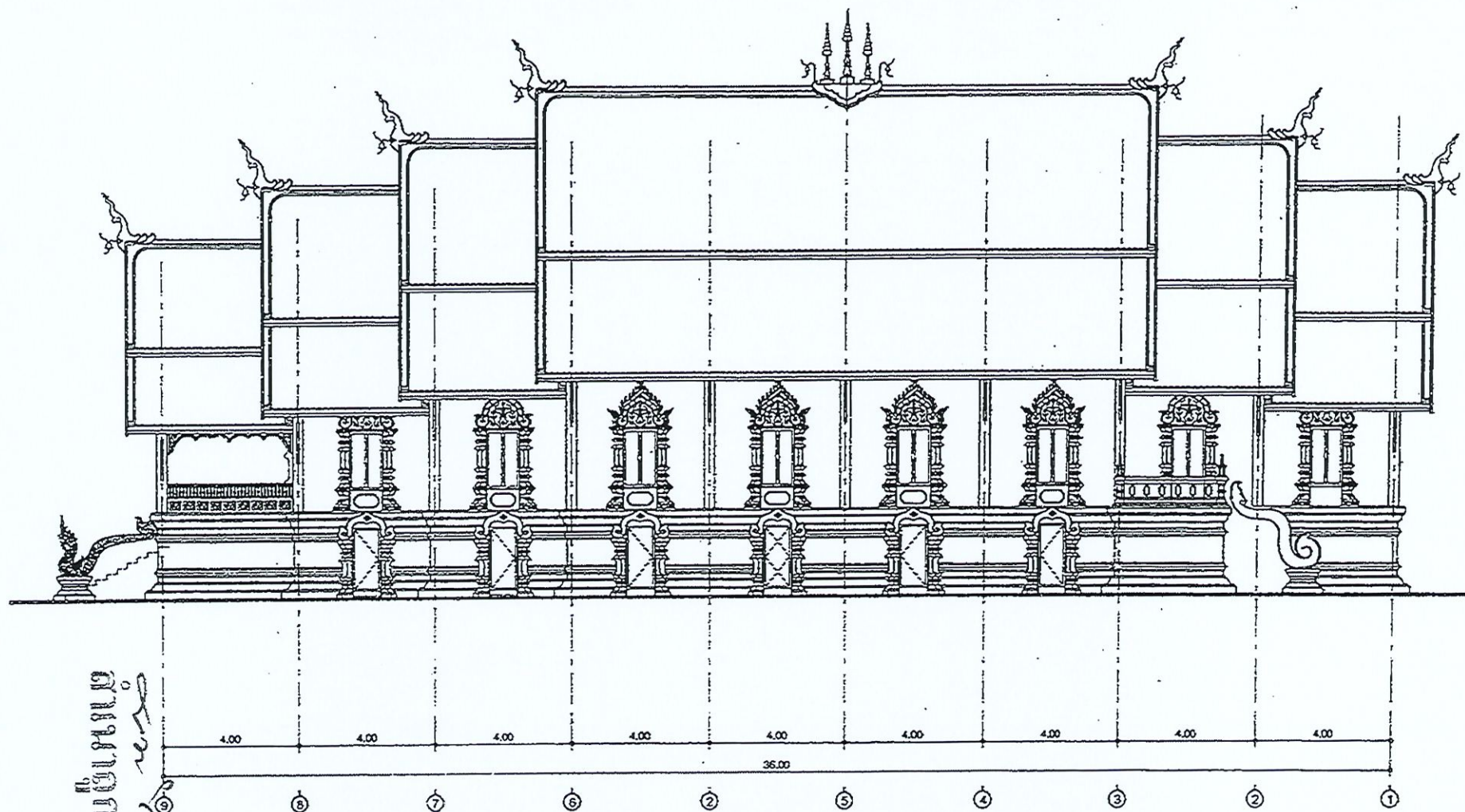
รูปตัดวิหาร - ด้านซ้าย มาตราส่วน 1:125
